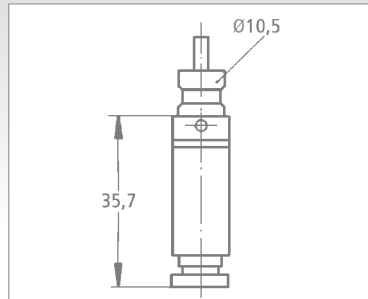
EV 25
