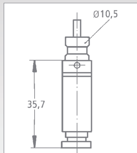
EV 35
