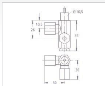
EV 3L
