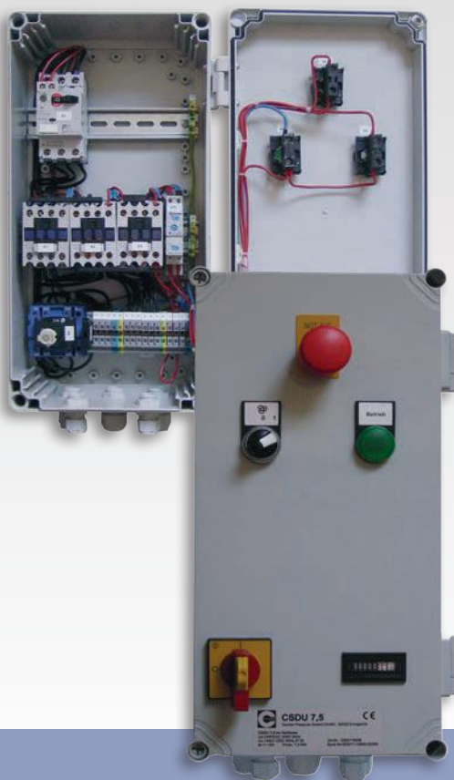
Fig. CSDU 7,5 complete
